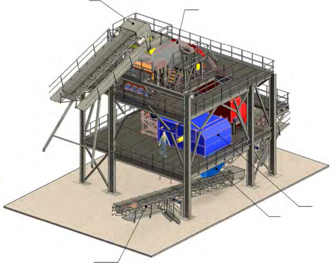
Комплекс СМС-1 (вид на узел сепарации) АО «Карельский окатыш» КСМС-800 на основе БС-Л-90/250-Н-21.127
