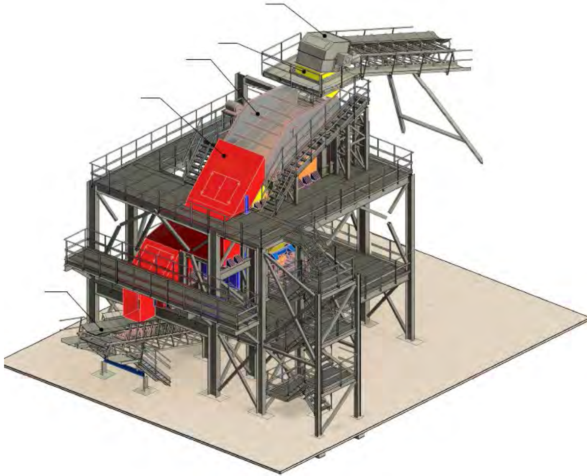
Комплекс СМС-1 (вид на узел сепарации) АО «Карельский окатыш» КСМС-800 на основе БС-Л-90/250-Н-21.127
