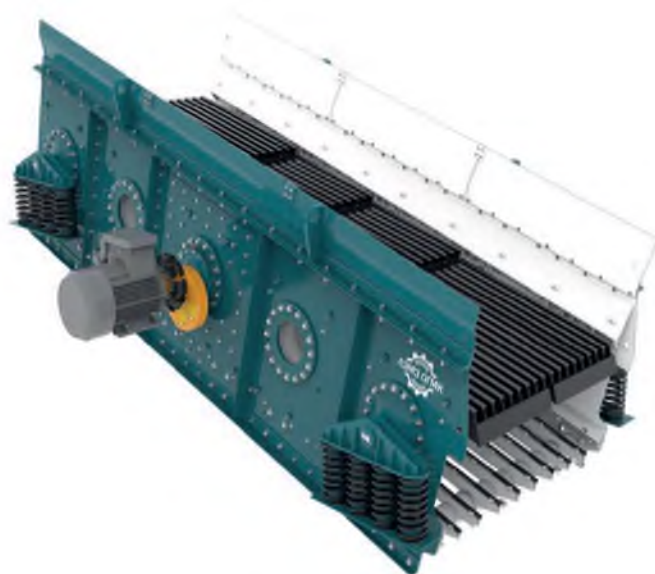
Одноярусный грохот
